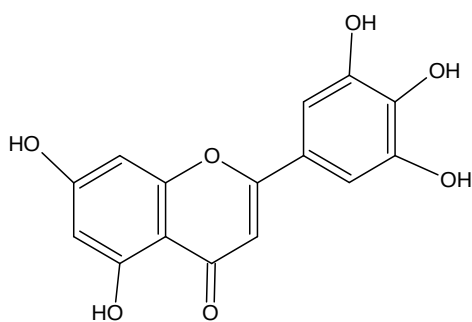
(32) Tricetin
