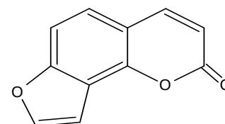
(25) Angélocine
